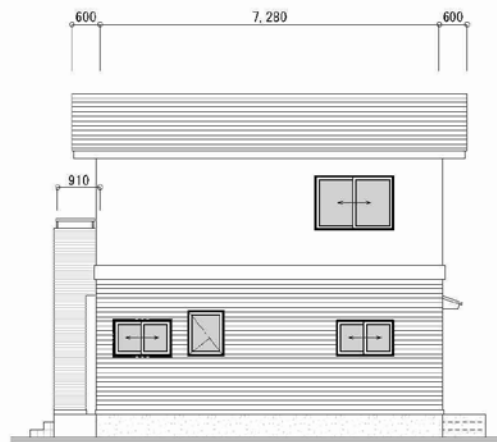
C案南立面図 1:100
