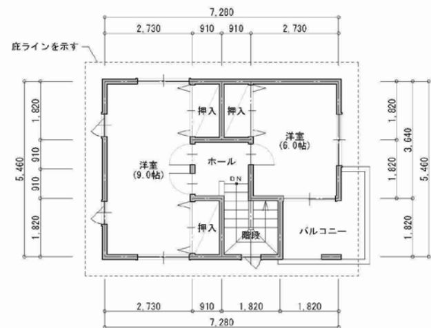
C案2階平面図 1:100
