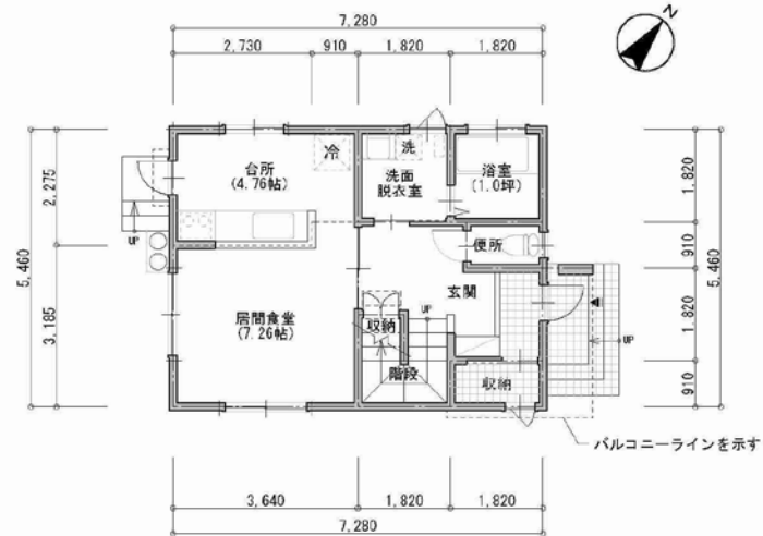
C案1階平面図 1:100
