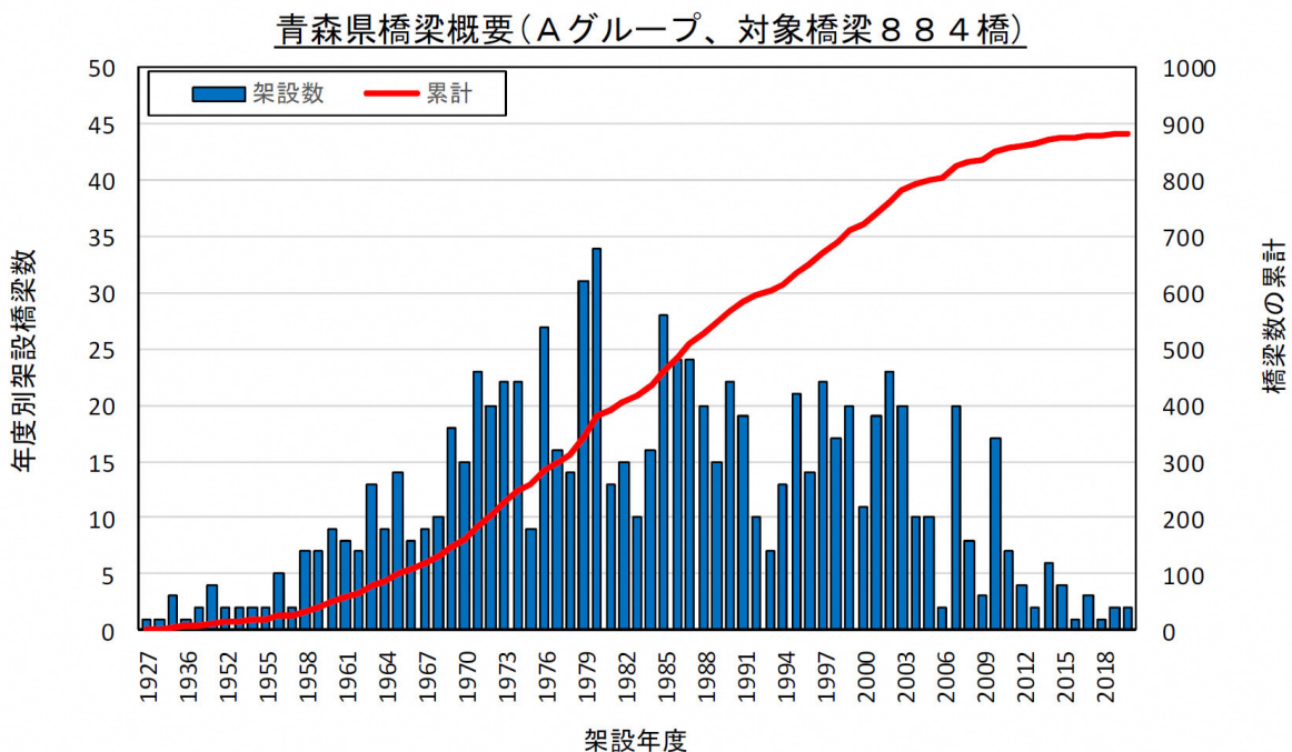
図 1-1 Aグループ橋梁の供用年度分布
