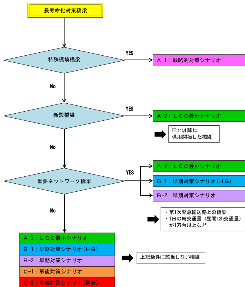
図5-6 維持管理シナリオ候補の選定フロー
