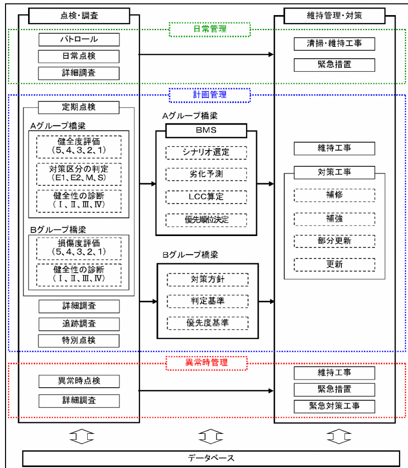
図5-1 維持管理体系
