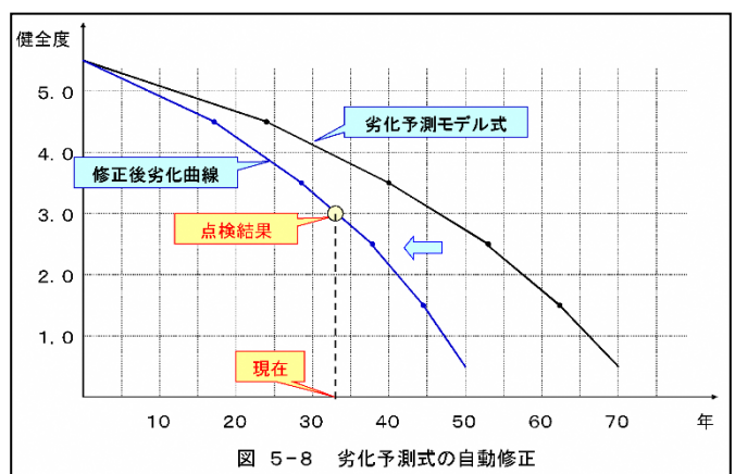
図 5-8 劣化予測式の自動修正
