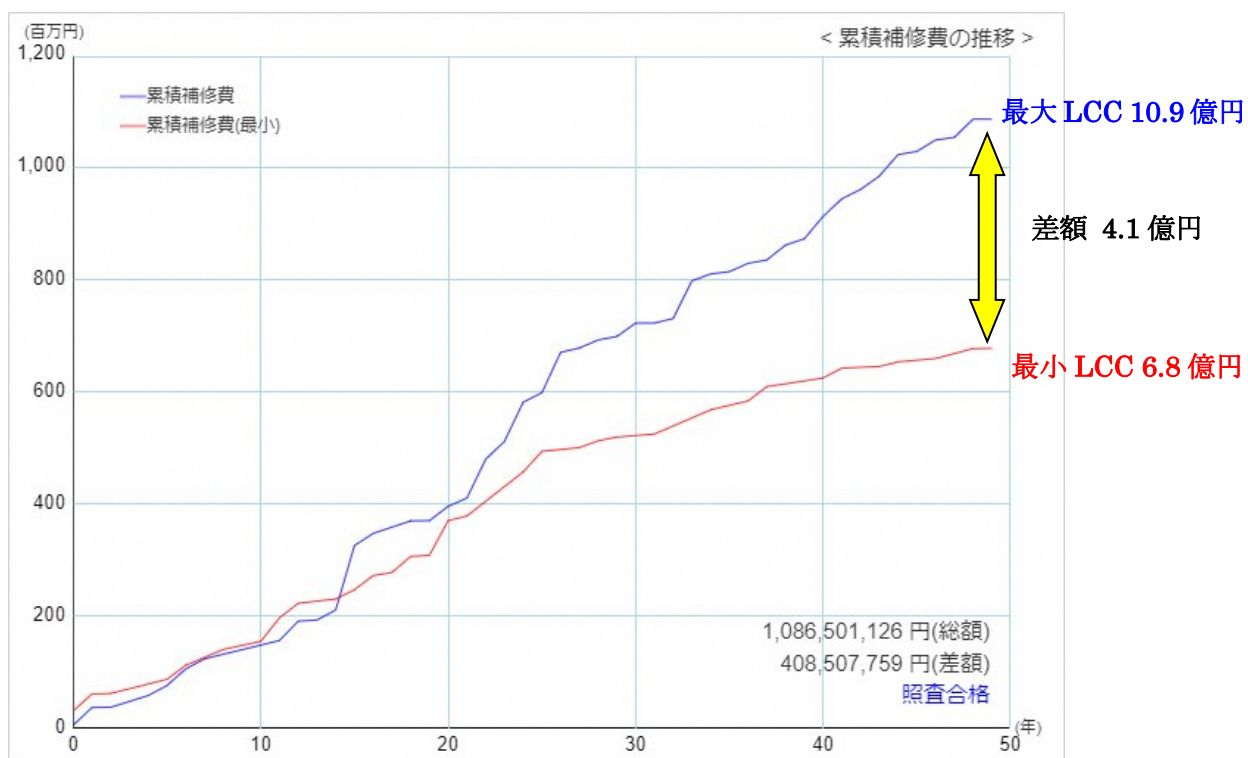
図 5-11 全橋梁の LCC 算定結果
