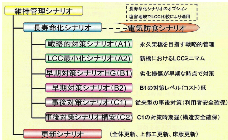
図5-5 維持管理シナリオ
