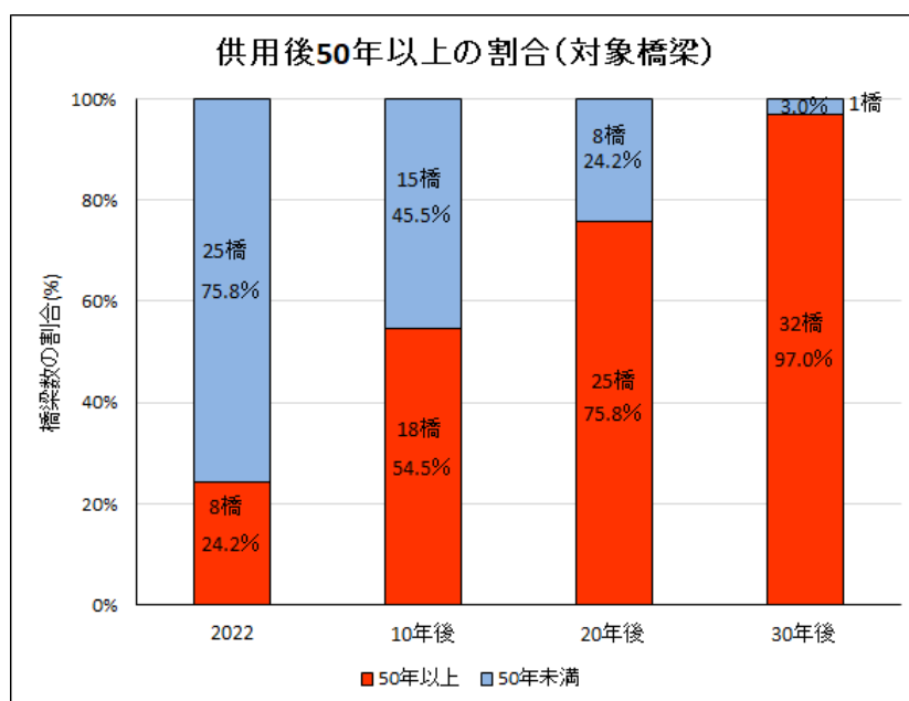
図3-1 供用後50年以上の割合
