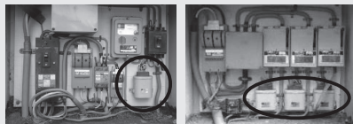
低圧分電盤内の低圧コンデンサー
